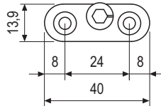
Regolazione perno
