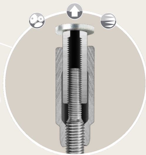
Sistema de embolo con doble rosca.
